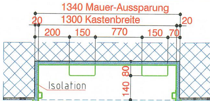
Grundriss Oberseite
