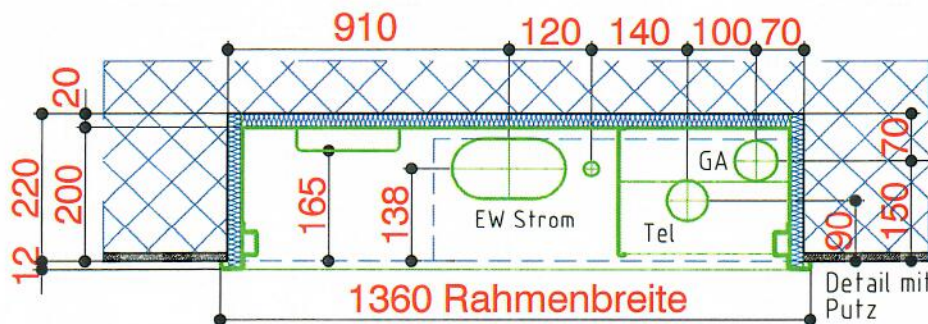
Grundriss Unterseite
