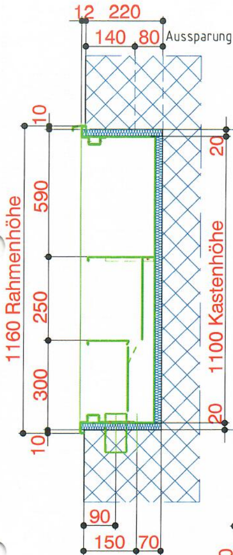
Vertikalschnitt
