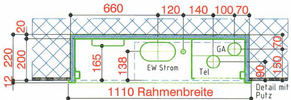
Grundriss Unterseite
