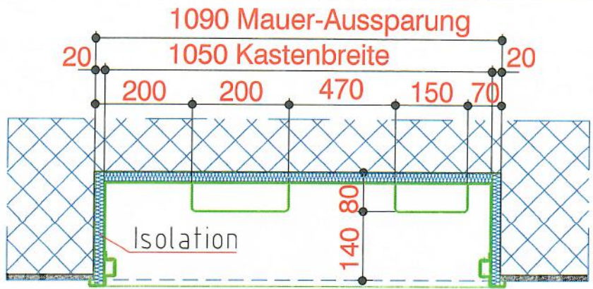
Grundriss Oberseite
