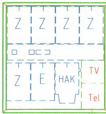
Grundriss Unterseite
