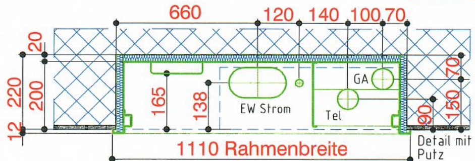
Grundriss Unterseite
