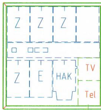
Grundriss Unterseite
