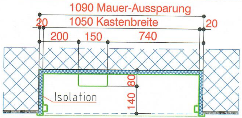
Grundriss Oberseite
