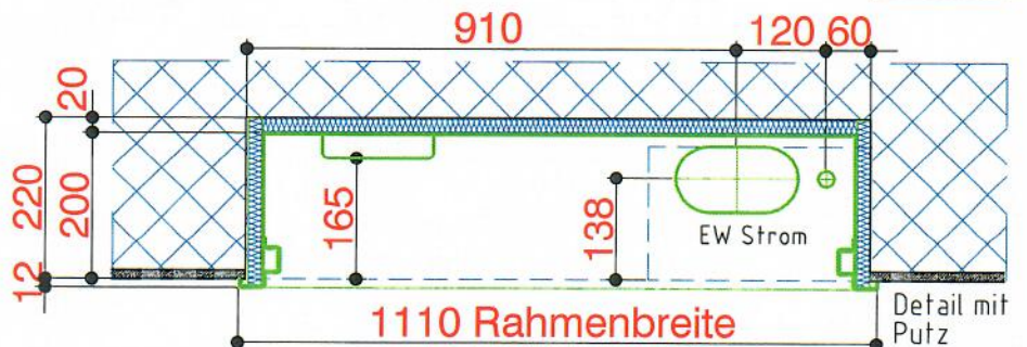
Grundriss Unterseite
