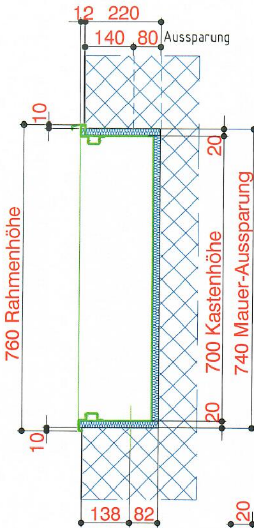
Vertikalschnitt
