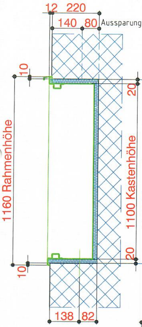
Vertikalschnitt
