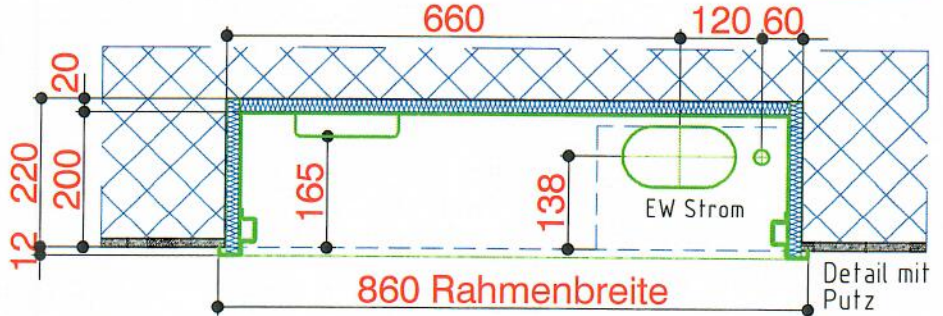
Grundriss Unterseite
