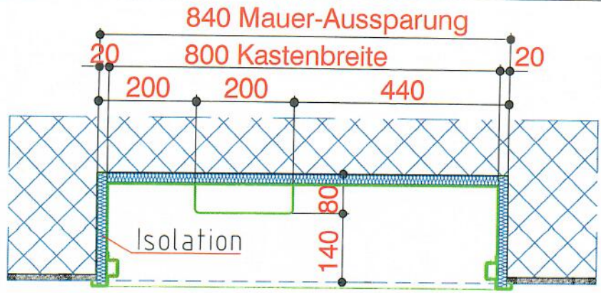
Grundriss Oberseite
