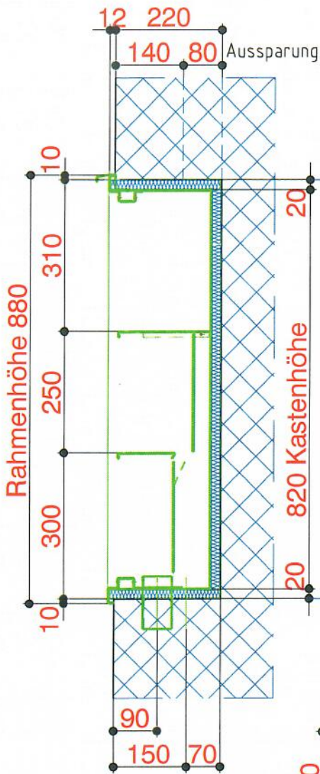
Vertikalschnitt
