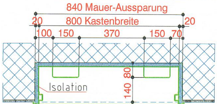
Grundriss Oberseite
