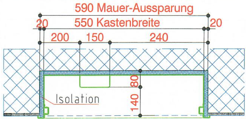
Grundriss Oberseite
