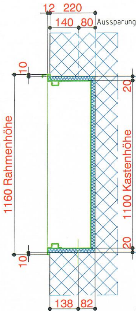
Vertikalschnitt
