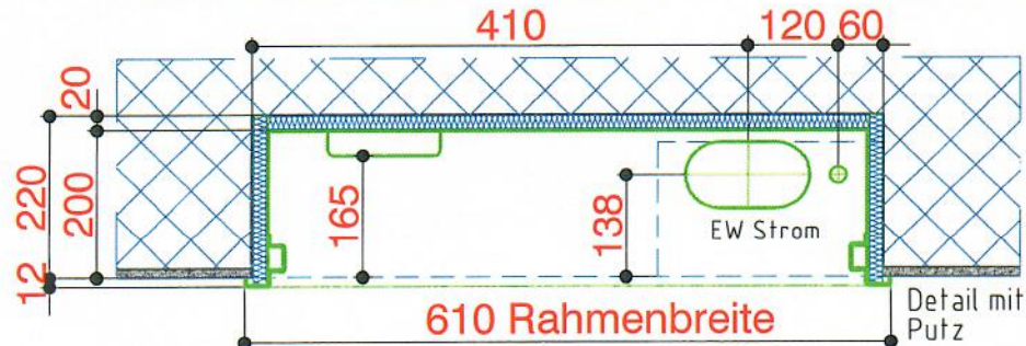
Grundriss Unterseite
