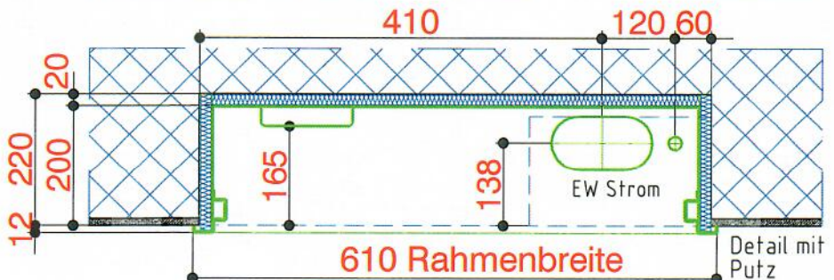
Grundriss Unterseite
