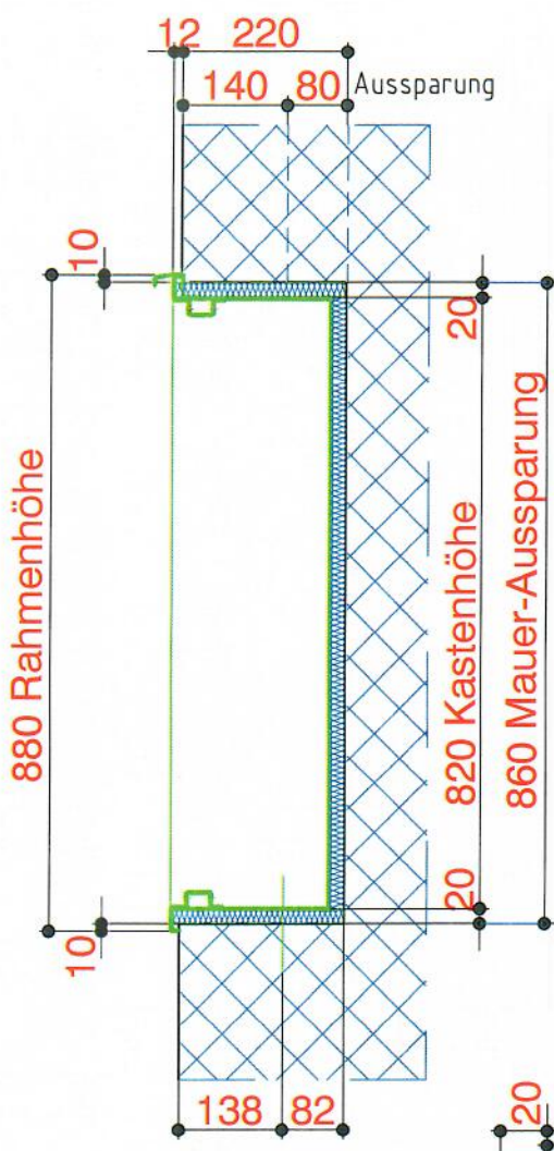
Vertikalschnitt
